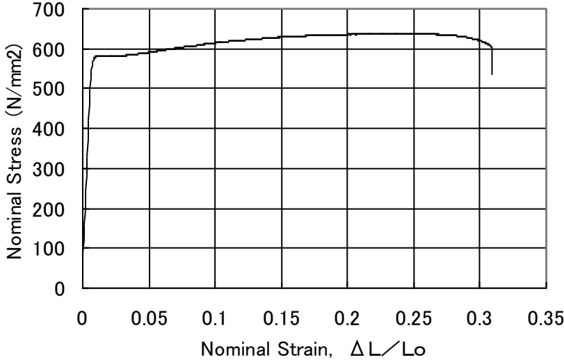
S-S curve (temper H, longitude to rolling)
