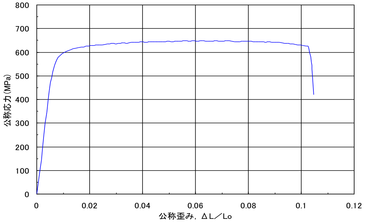
図 13 C7025-TR02 の圧延平行方向の S-S カーブ
